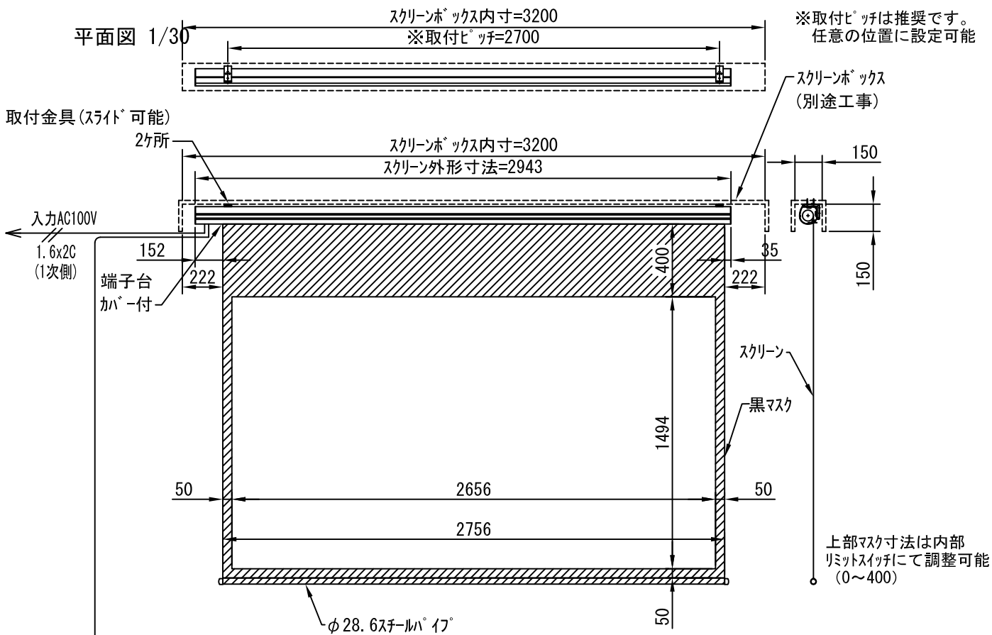
外観図 1/30
