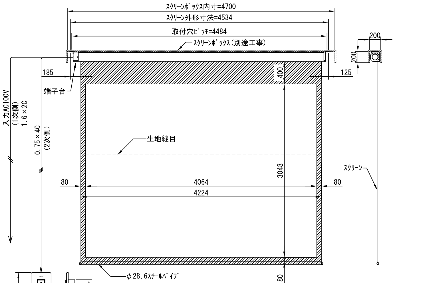
外観図 1/40
