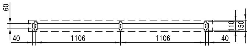
平面図 1/30
