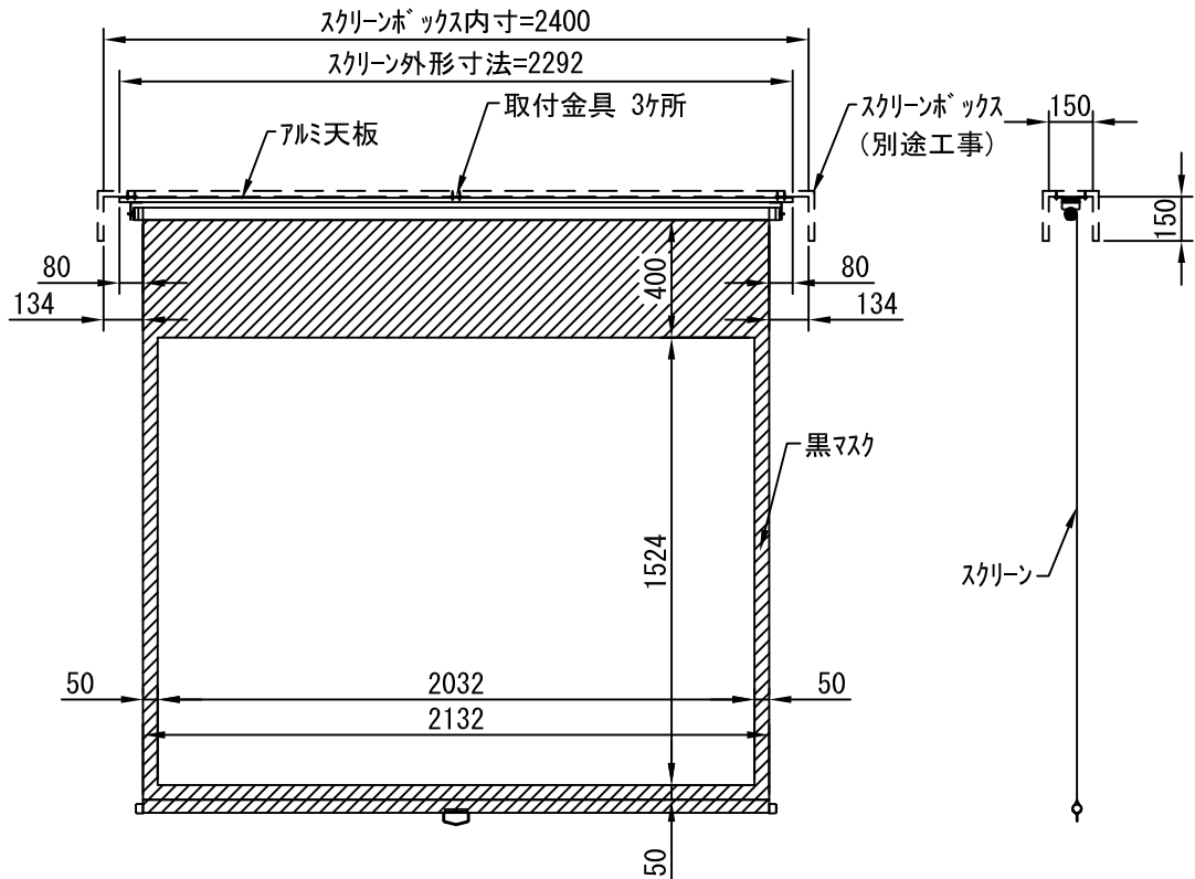
正面図 1/30
